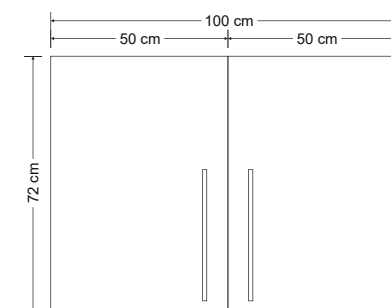
HS 100 - esquisse
