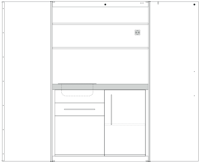
esquisse: SKM - Modèle de base sans appareils
