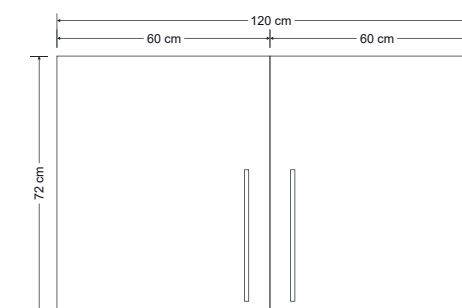
HS 120 - esquisse
