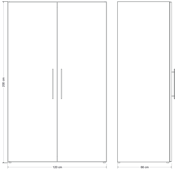
esquisse: SKM - Dimensions
