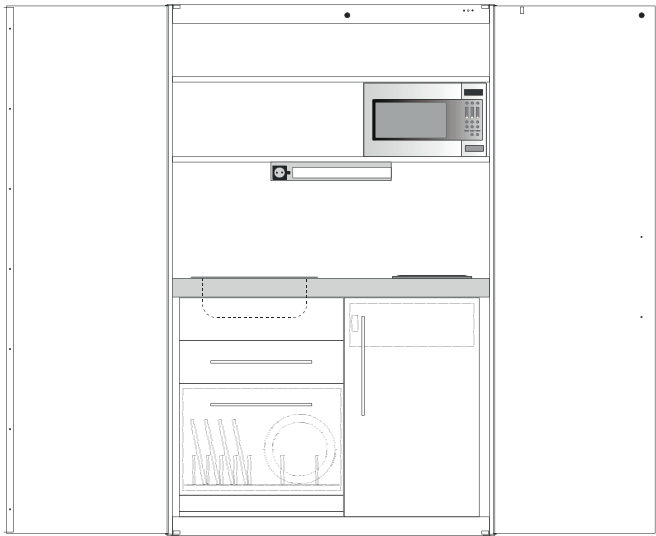
esquisse: SKM - avec équipement complet
