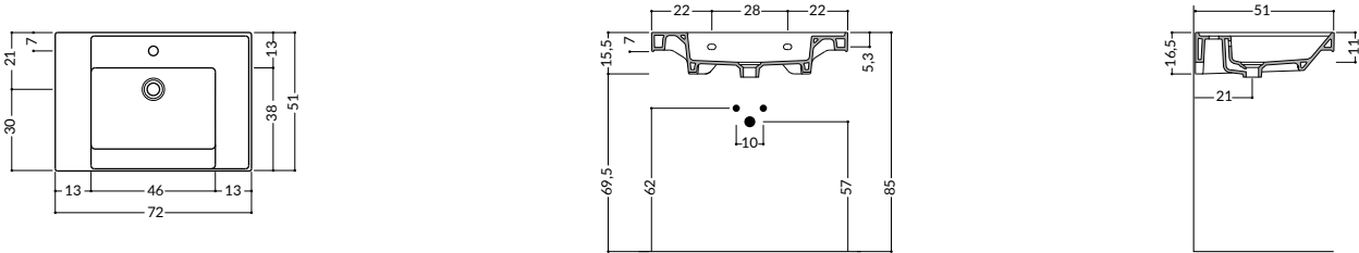
Vera 92 - 92x51 H11 cm - Kg 27
