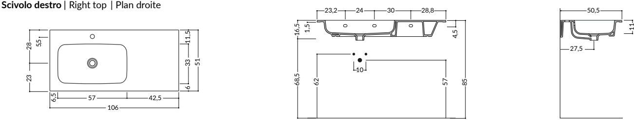
Zulu 121 - 121x51 H1,5 cm - Kg 39 Vasca centrale | Central basin | Cuve centrale
