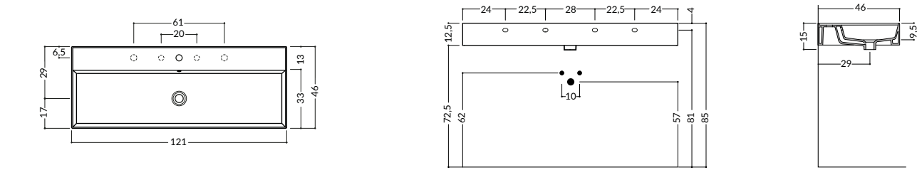
Lira 121 - 121x46 H12,5 cm - Kg 33 Vasca centrale | Central basin | Cuve centrale
