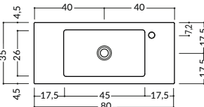
Slim 80 - 80x35 H5 cm - Kg 16
