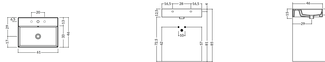
Lira 61 - 61x46 H12,5 cm - Kg 18 Vasca destra | Right basin | Cuve droite Scivolo sinistro | Left top | Plan gauche
