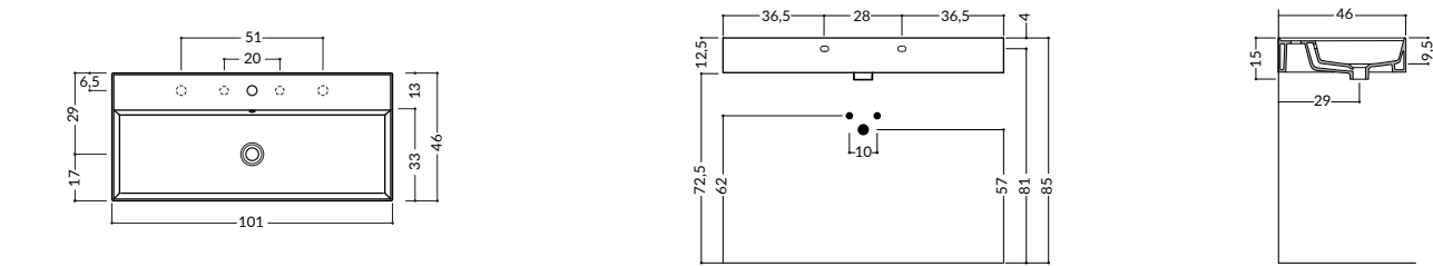
Lira 101 - 101x46 H12,5 cm - Kg 27 Vasca destra | Right basin | Cuve droite Scivolo sinistro | Left top | Plan gauche
