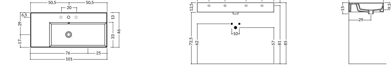
Lira 101 - 101x46 H12,5 cm - Kg 27 Vasca sinistra | Left basin | Cuve gauche Scivolo destro | Right top | Plan droite
