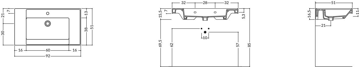
Vera 107 - 107x51 H11 cm - Kg 30
