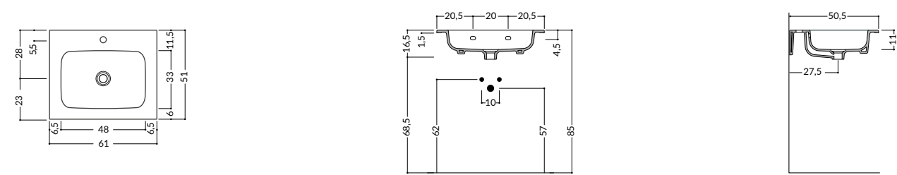
Zulu 71 - 71x51 H1,5 cm - Kg 19
