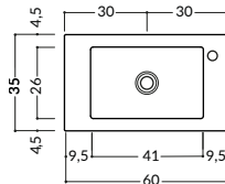
Slim 60 - 60x35 H5 cm - Kg 12
