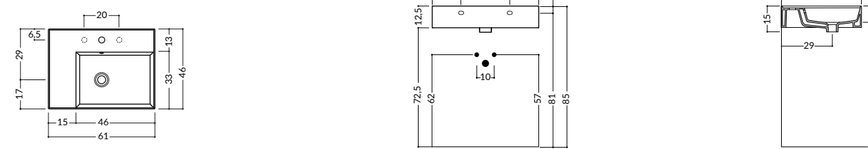
Lira 61 - 61x46 H12,5 cm - Kg 18 Vasca sinistra | Left basin | Cuve gauche Scivolo destro | Right top | Plan droite
