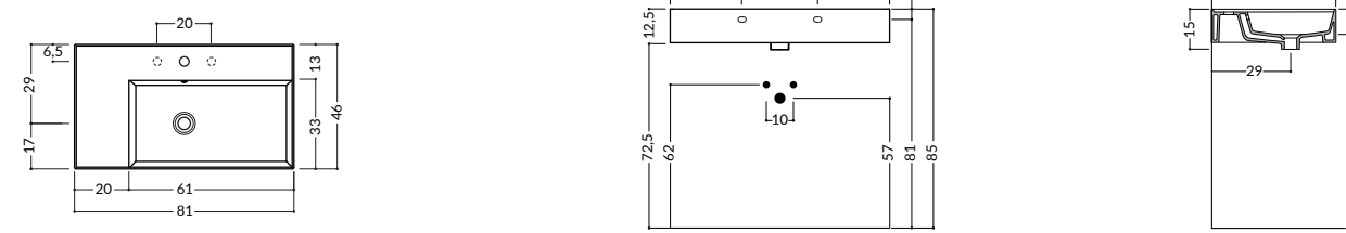
Lira 81 - 81x46 H12,5 cm - Kg 21 Vasca destra | Right basin | Cuve droite Scivolo sinistro | Left top | Plan gauche
