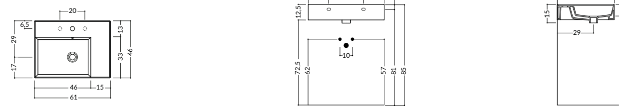
Lira 81 - 81x46 H12,5 cm - Kg 20 Vasca centrale | Central basin | Cuve centrale
