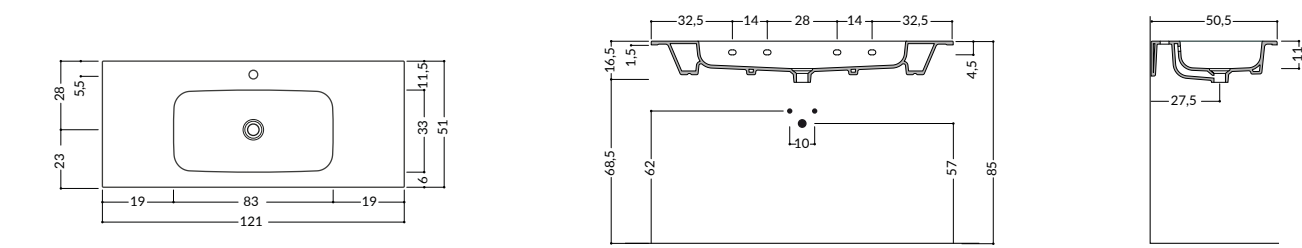
Zulu 121 - 121x51 H1,5 cm - Kg 37
