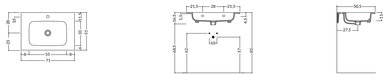
Zulu 91 - 91x51 H1,5 cm - Kg 26
