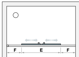
FOP2 reversibile Reversible FOP2 - FOP2 réversible
