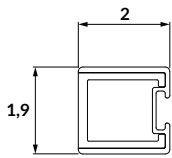
Profilo di battuta per versione a nicchia (BLP4). Deflection profile for niche (BLP4). Profilé de butée pour niche (BLP4).
