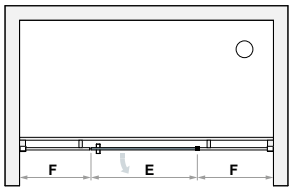
TIP7 DX - TIP7 Rh - TIP7 D
