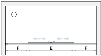
STP2 reversibile Reversible STP2 - STP2 réversible
